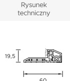
Próg PVC z uszczelką Premium Termo
