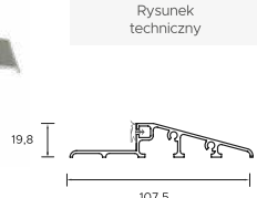
Próg aluminiowy z uszczelką Premium, Normal, Protect, Iron do ościeżnicy "9" (kątownej), "11" (wewnętrznej)
