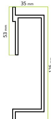
przekrój
