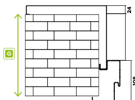
Rysunek techniczny
