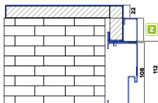
Ościeznica Alu Hybrid
